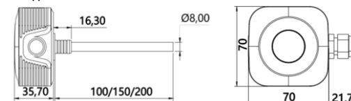
Размеры датчика, мм
