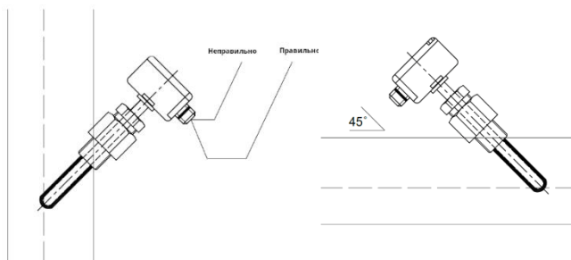
Схемы установки для вертикальной и горизонтальной трубы
