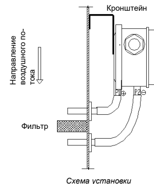
Схема установки
