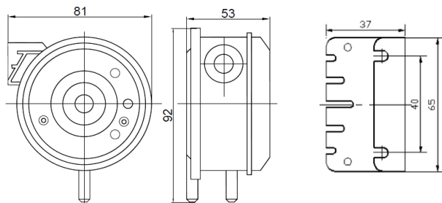
Габаритные и установочные размеры, мм
