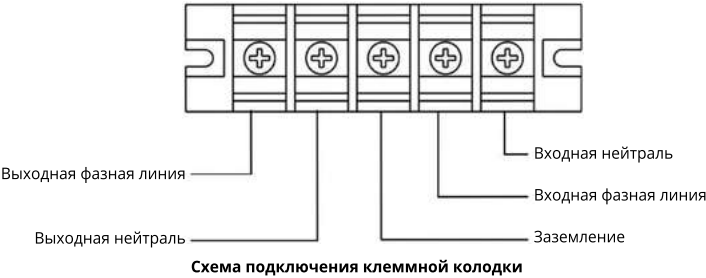
Схема подключения клеммной колодки
