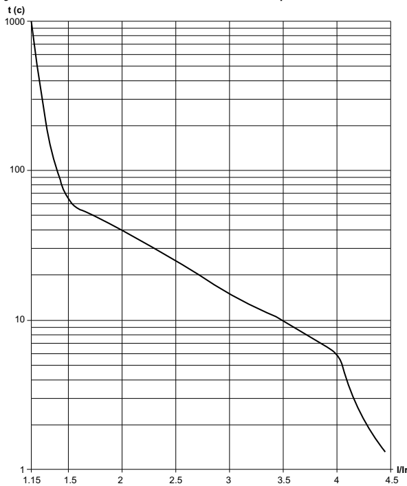
Времятоковая кривая защиты стартера от перегрузки
