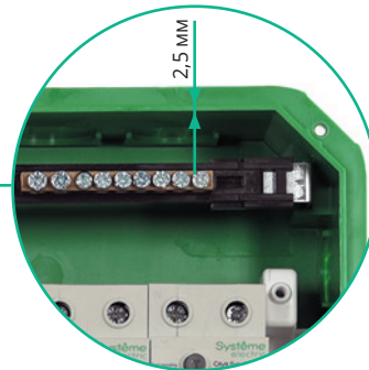
Жесткость конструкции
