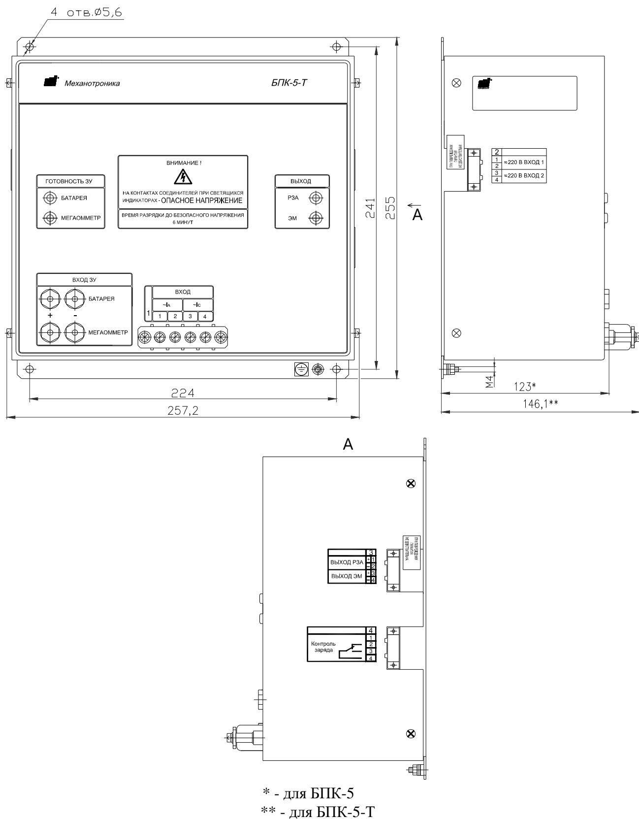
Рисунок 1 - Габаритные и установочные размеры БПК
