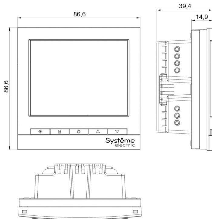
Габаритные размеры комнатного термостата RTF4VIML
