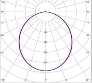
Кривая силы света: Рисунок 1
