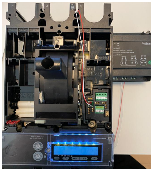
Итоговая фотография для автомата 630A / Final image for CCB 630A
