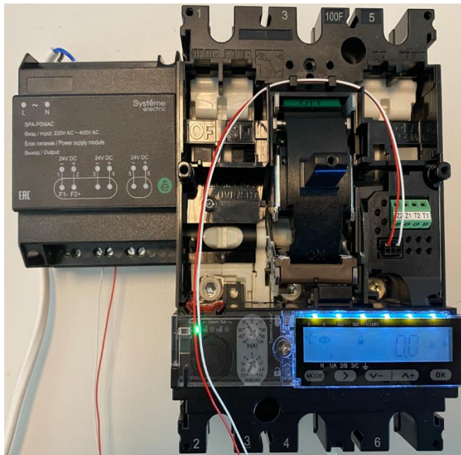
Итоговая фотография для автомата 250A / Final image for CCB 250A
