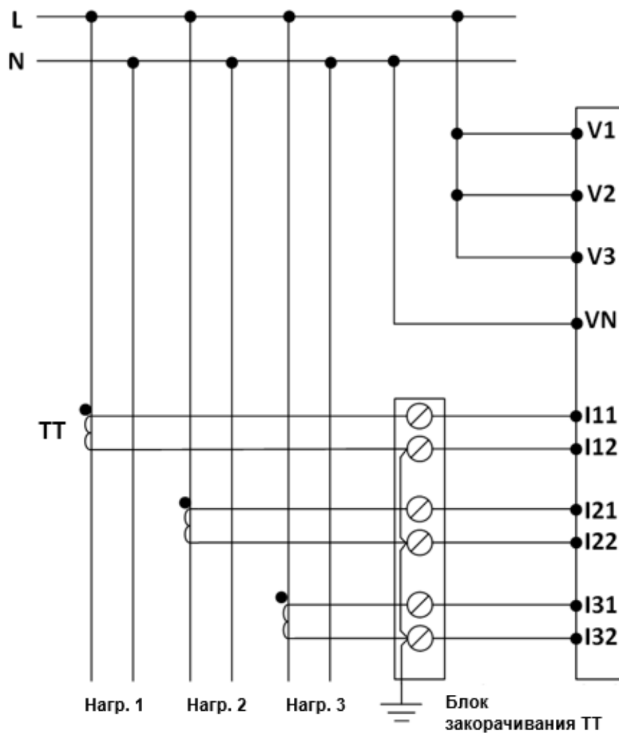
Рисунок 3.4.10 3x1Ф прямое подключение (3 ТТ)
