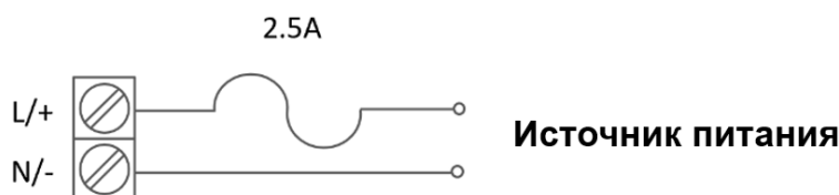
Рисунок 3.10 Подключение входов питания
